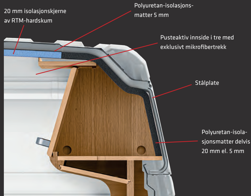
Malibu Van: gjennomarbeidede isoleringstiltak for karosseriet
