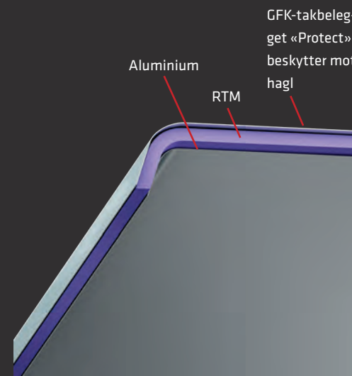
Malibu Van hybrid-hevetak med klassens beste isolasjonskonsept i sandwichkonstruksjon og med lav egenvekt
