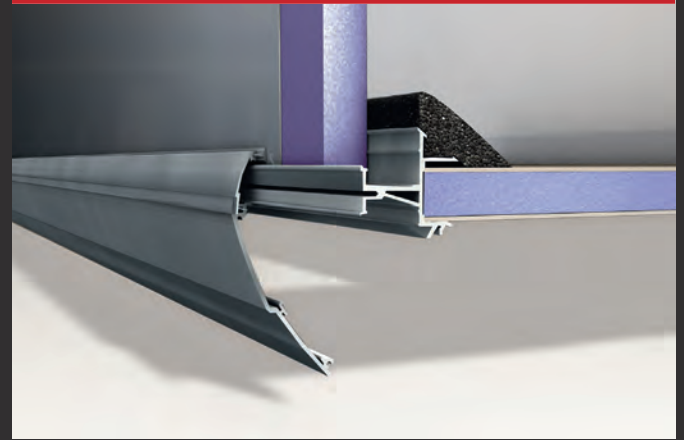
3 Hopsättningen sidovägg/golv görs med mycket stabil balk
