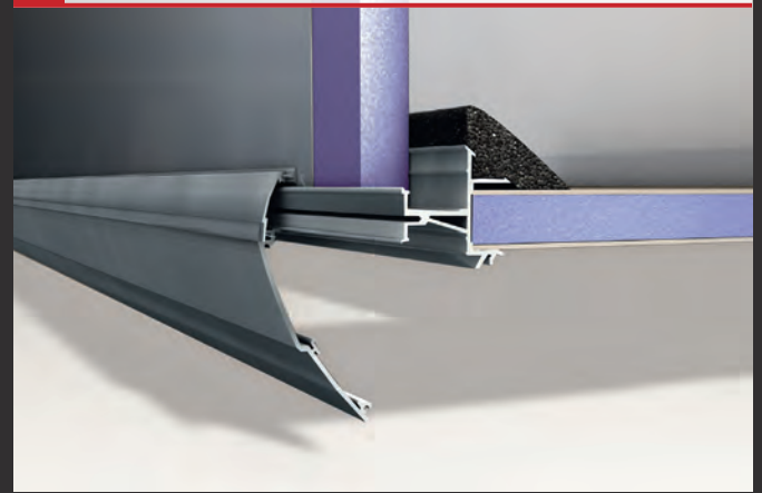
3 Forbindelse sidevegg/gulv via høystabil bærebjelke
